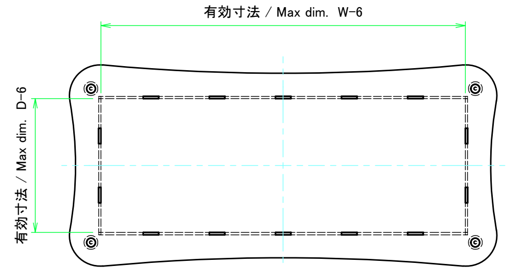
下カバー / Bottom cover
